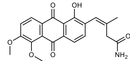
Kianthraquinone
